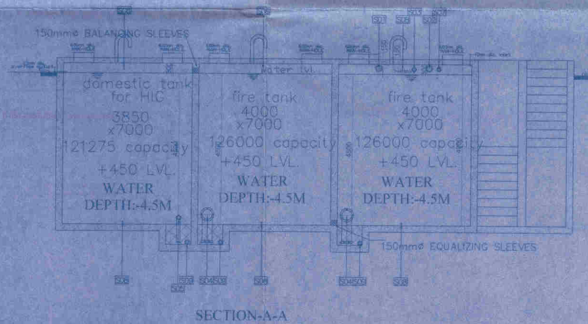
UGR PLAN & SECTION
